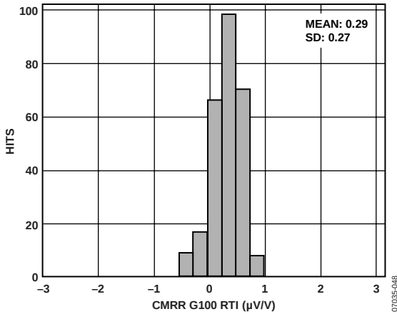
图7. CMRR典型分布图( G = 100 )
