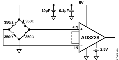
图49. 精密应变计
