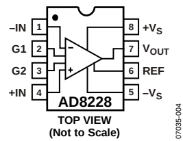
图2. 引脚配置
