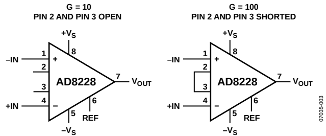
图42. 设置增益
