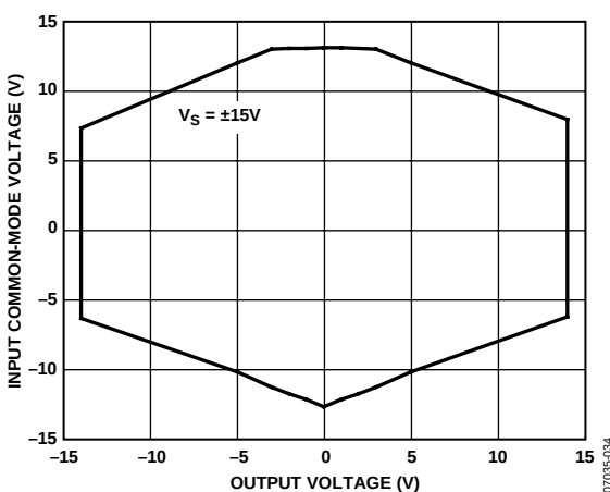
图11. 输入共模电压与输出电压的关系 ( V_S = \pm 15V , G=10 )
