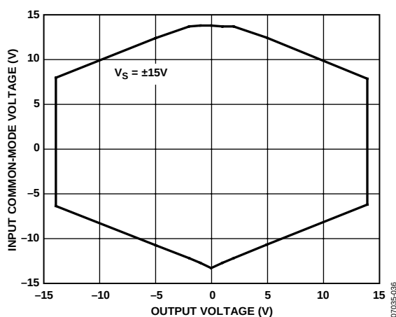
图13. 输入共模电压与输出电压的关系 ( V_S = \pm 15V , G=100 )
