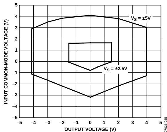
图12. 输入共模电压与输出电压的关系 ( V_S = \pm 2.5V , \pm 5V , G=100 )
