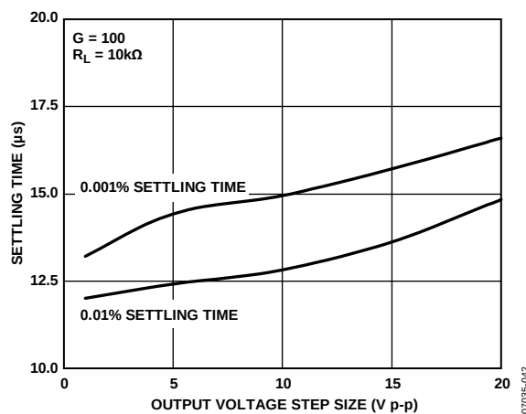
图40. 建立时间与阶跃大小的关系 ( G = 100 )
