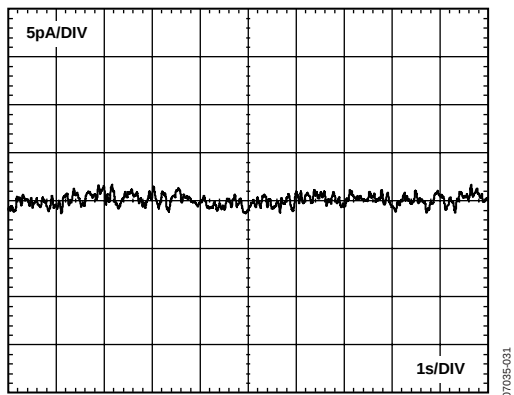
图33. 0.1 Hz至10 Hz电流噪声
