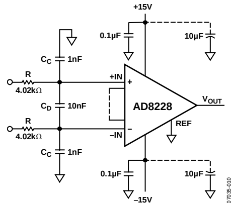
图47. 射频干扰(RFI)抑制
