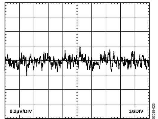
图31. 0.1 Hz至10 Hz折合到输入端电压噪声( G=10 )
