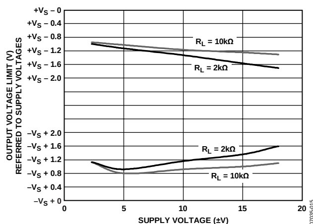
图25. 输出电压摆幅与电源电压的关系
