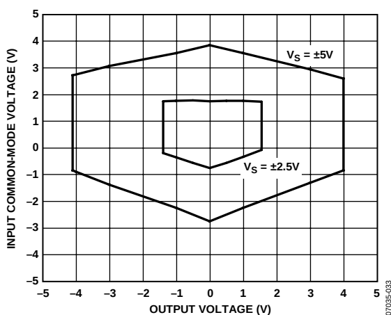
图10. 输入共模电压与输出电压的关系 ( V_S = \pm 2.5V , \pm 5V , G=10 )
