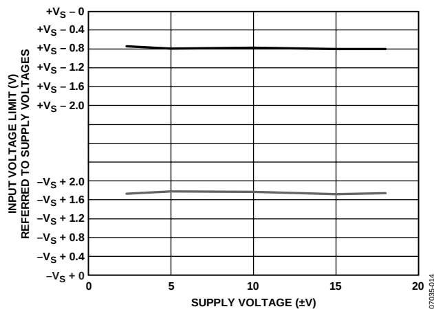
图24. 输入电压限制与电源电压的关系
