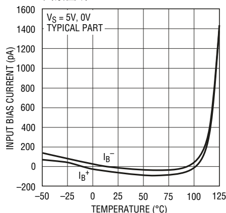
输入偏置电流与温度的关系曲线
