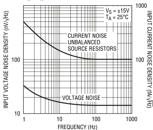
e_n 、 i_n 与频率的关系曲线
