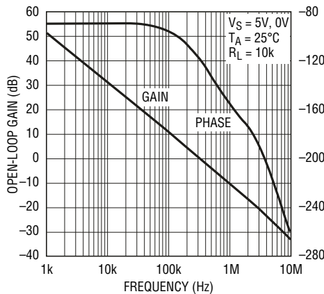
增益和相位与频率的关系曲线
