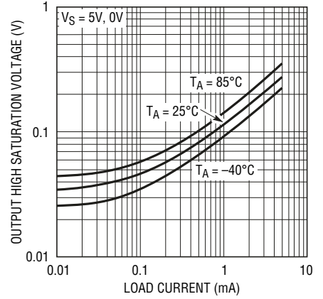
输出饱和电压与负载电流的关系曲线 (输出高)
