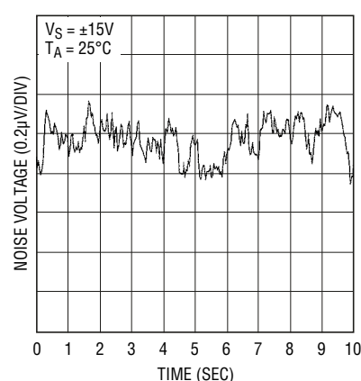
0.1Hz 至 10Hz 噪声
