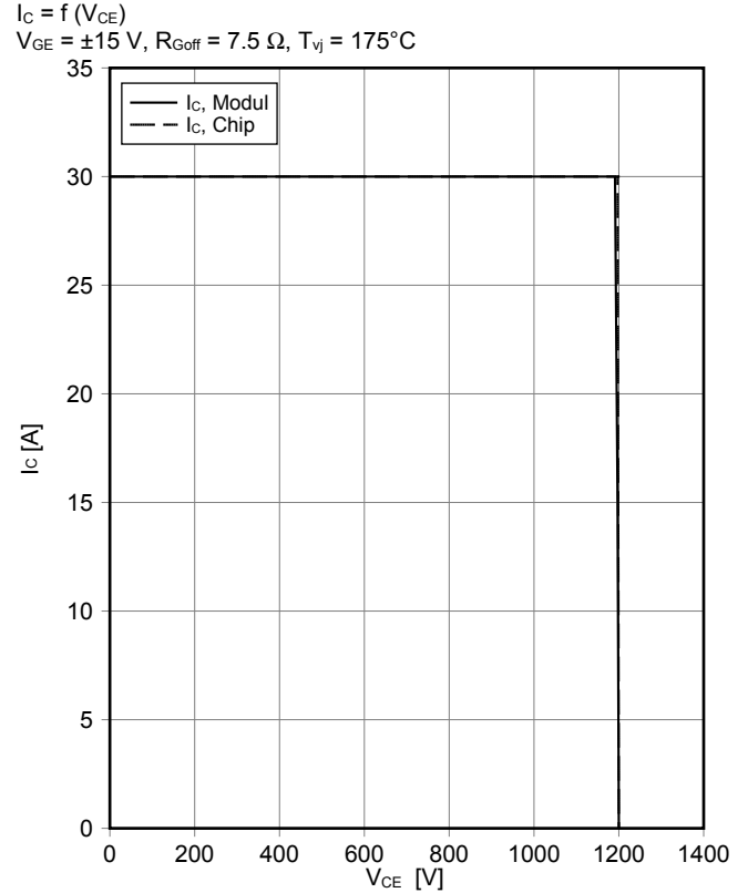
Sicherer Rückwärts-Arbeitsbereich IGBT, Wechselrichter (RBSOA) reverse bias safe operating area IGBT, Inverter (RBSOA) I_C = f(V_{CE}) V_{GE} = \pm 15\text{ V} , R_{Goff} = 7.5\ \Omega , T_{vj} = 175^\circ\text{C}
