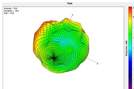
2450MHz
