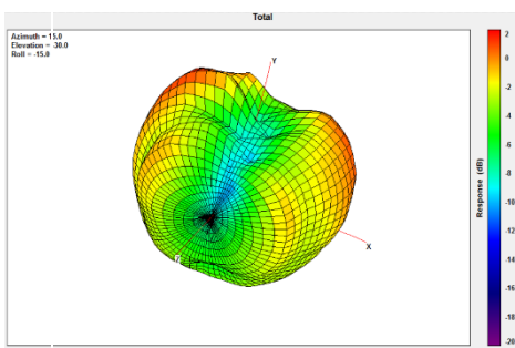
2400MHz
