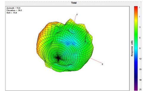
2500MHz
