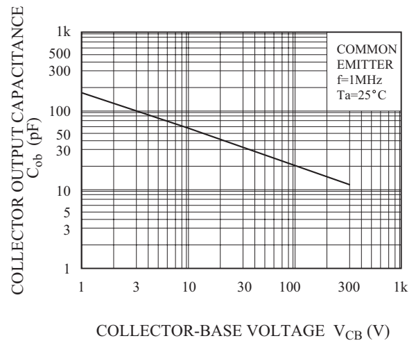
Fig 4. C_{ob} - V_{CB}
