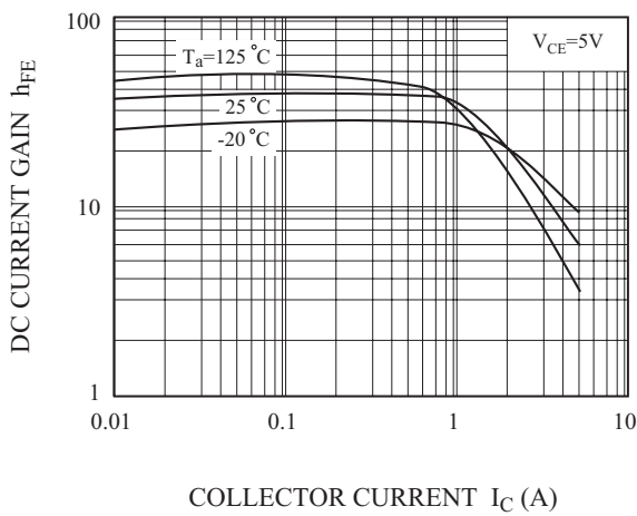
Fig 3. h_{FE} - I_C
