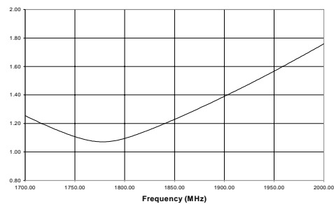
Input VSWR
