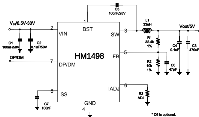
Fig. 1 Schematic
