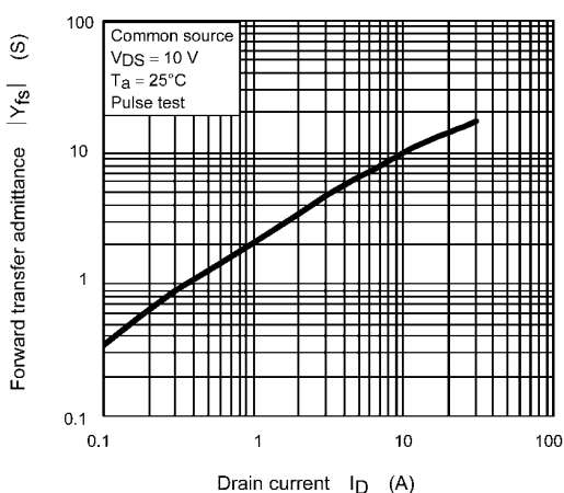
Fig. 8.5 |Y_{fs}| - I_D
