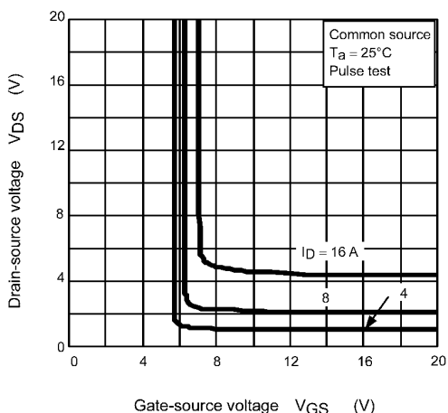
Fig. 8.4 V_{DS} - V_{GS}
