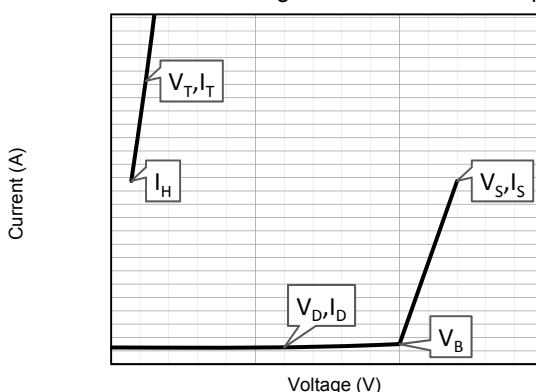
Fig.4 - VI Curve
