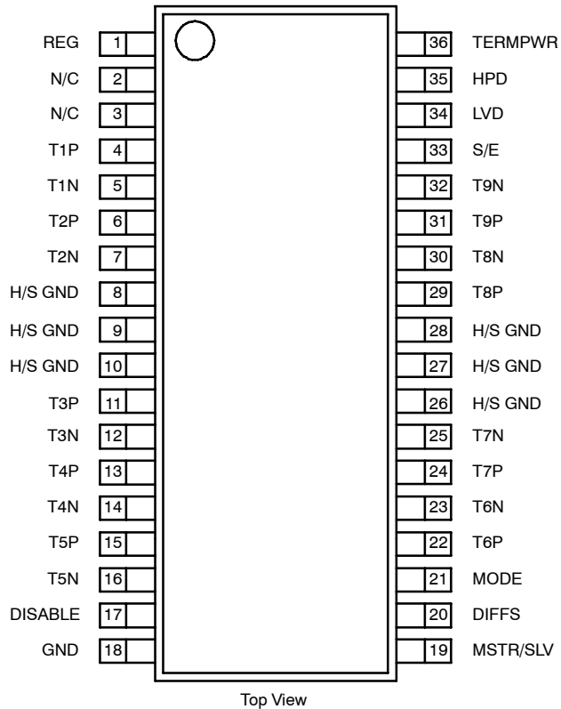
SiP5630 (QSOP-36)
