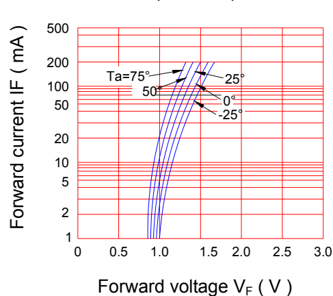
I_F vs. V_F
