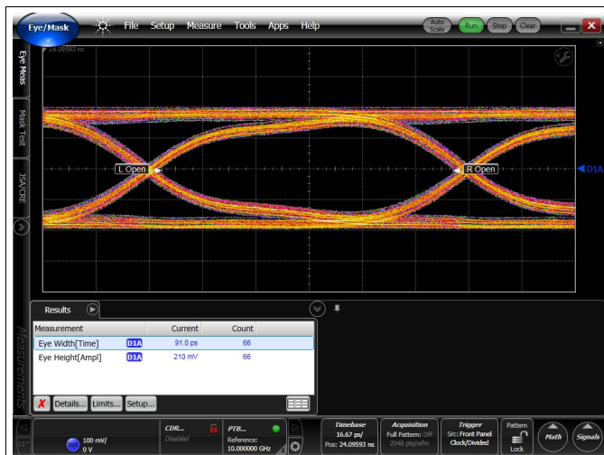
图 10. Source 10 Gbps Eye Diagram
