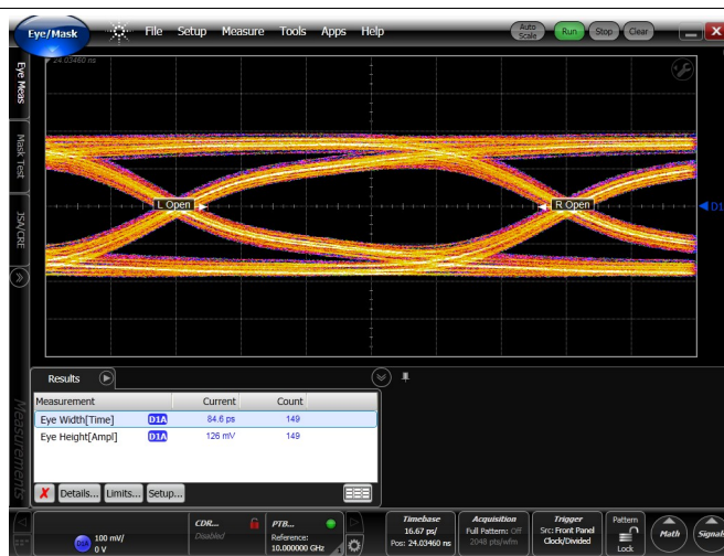
图 11. HD3SS3202 10 Gbps Output Eye Diagram
