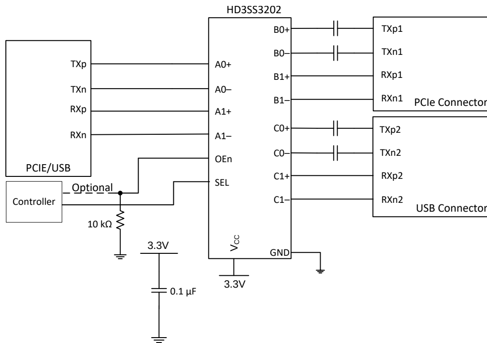
图 13. PCIE Motherboard
