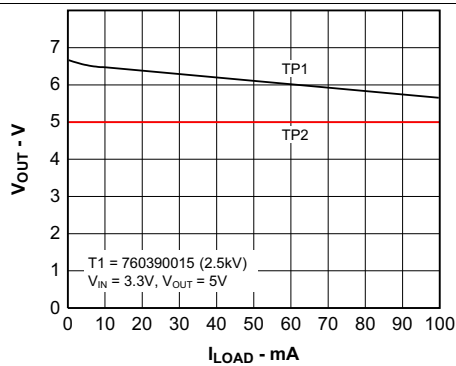
图 9. Output Voltage vs Load Current
