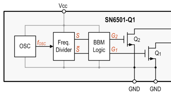
图 39. SN6501-Q1 Block Diagram
