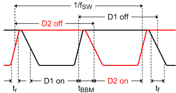
图 34. Timing Diagram
