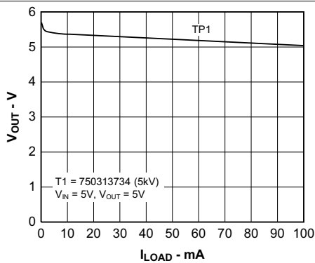
图 15. Output Voltage vs Load Current
