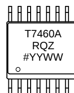
QSOP-16 CASE 492
