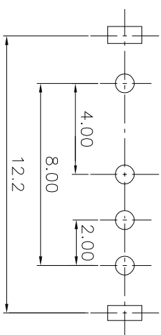
P.C.B layout
