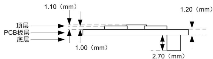
图 6.3 RS200 高度尺寸
