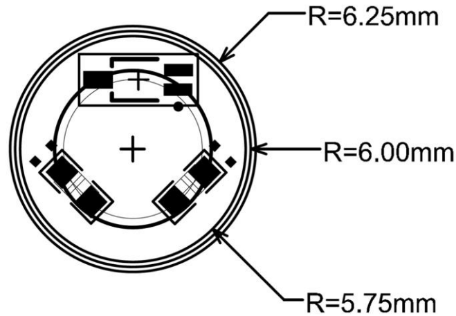
图 6.1 RS200 正面尺寸
