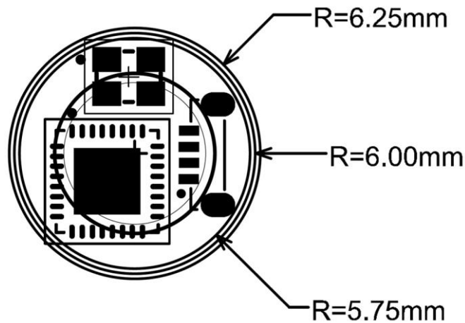
图 6.2 RS200 背面尺寸
