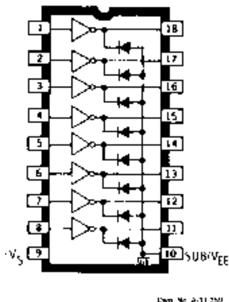
UDN2580A and UDN2585A
