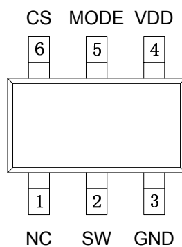
SOT23-6
