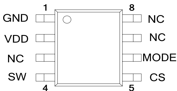
ESOP8
