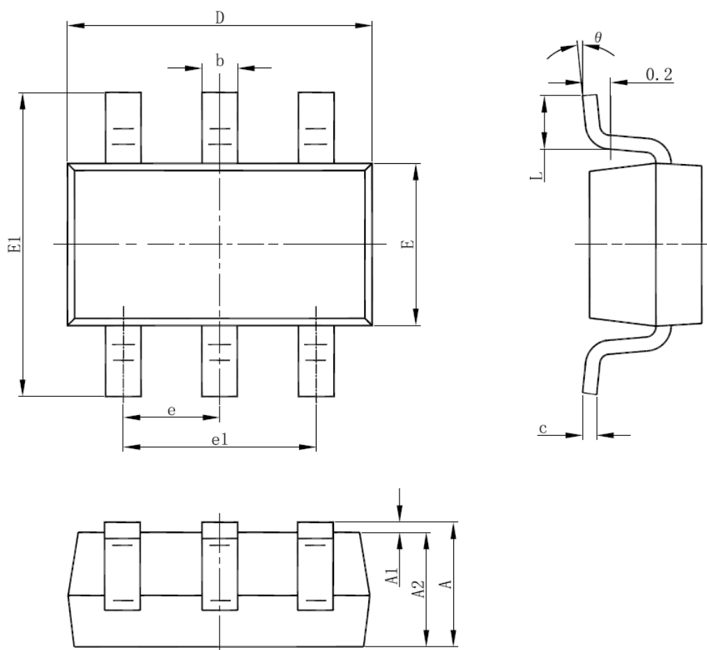
SOT23-6 封装尺寸图:
