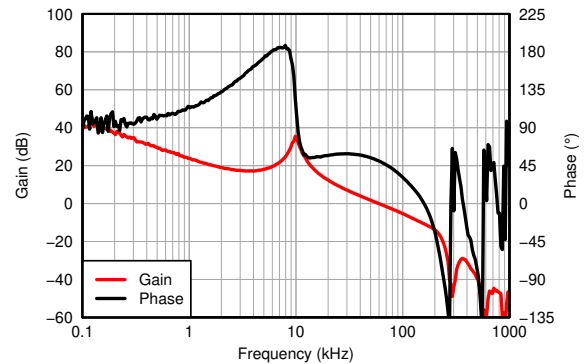
图 7-3. Loop Response
