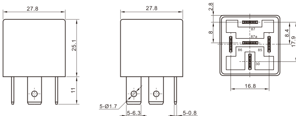
外形尺寸 Outline Dimensions
