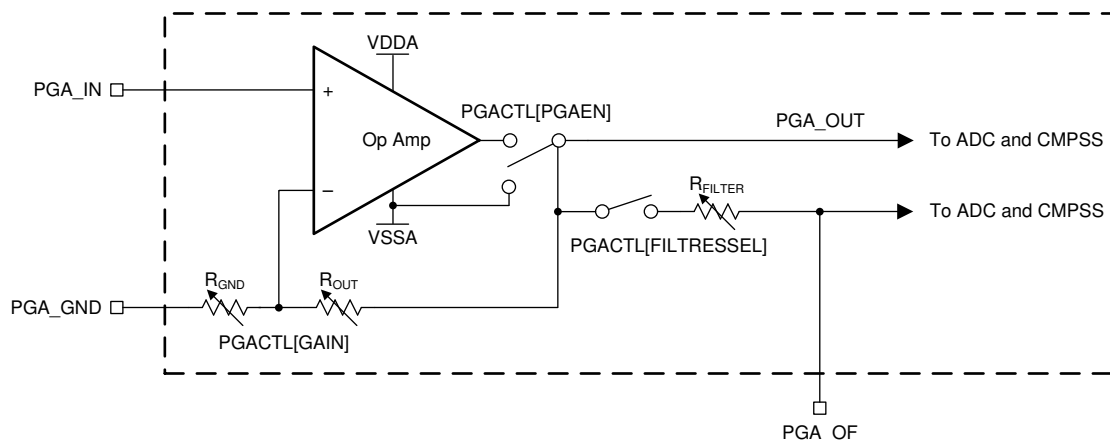
图 7-45. PGA 方框图
