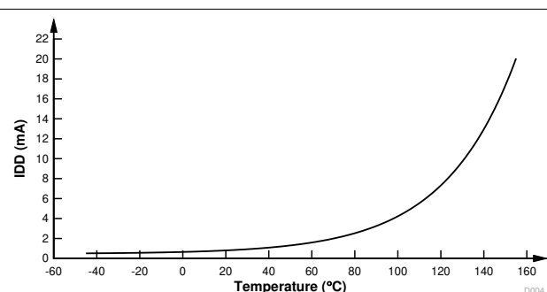
图 7-5. Halt 电流与温度间的关系 (°C)
