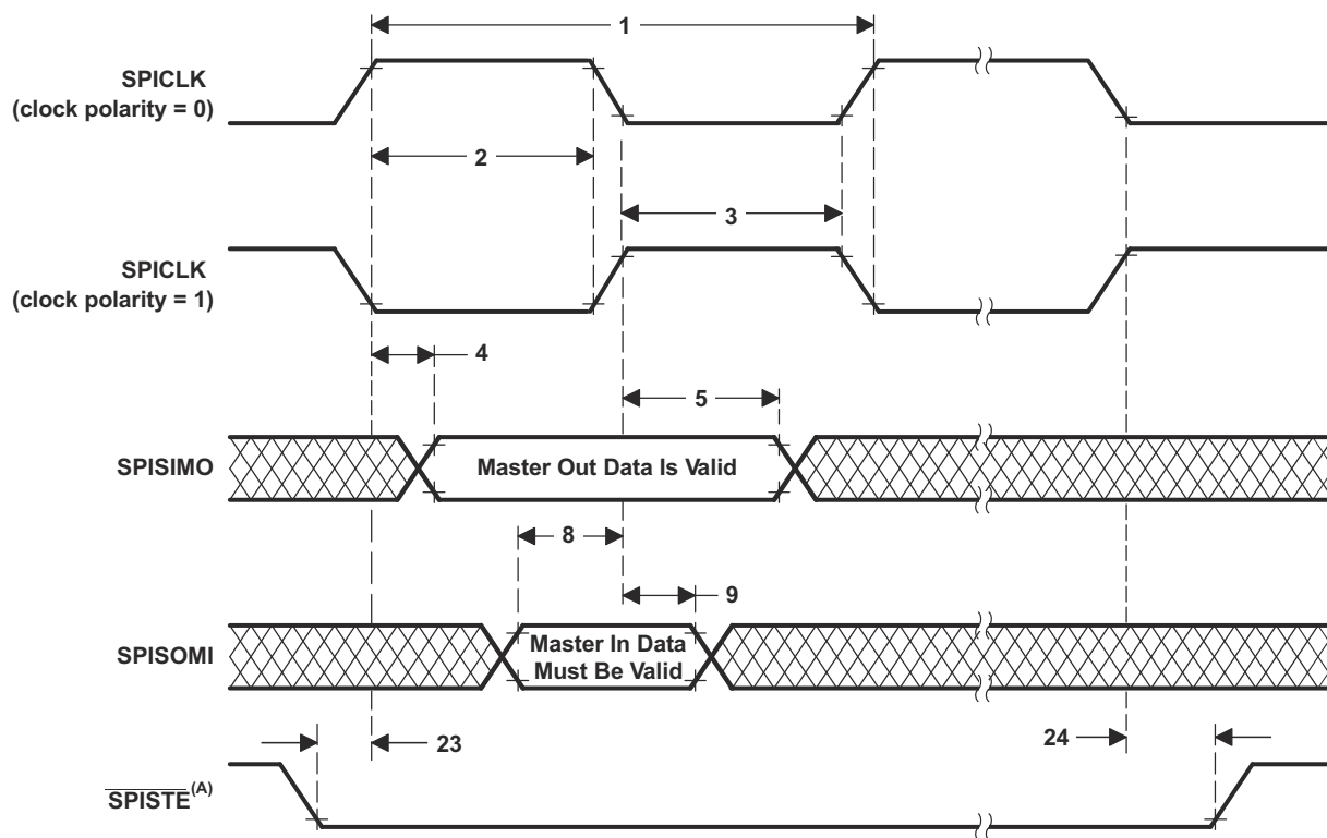
图 7-88. 高速 SPI 主模式外部时序 (时钟相位 = 0)
