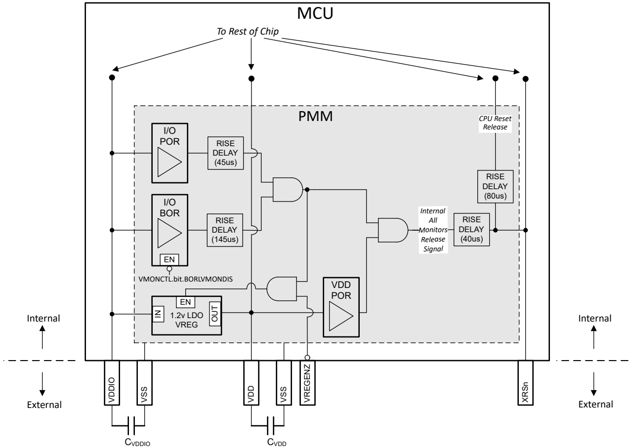
图 7-6. PMM 方框图
