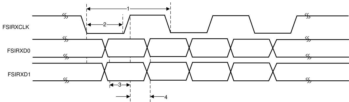
图 7-98. FSIRX 时序
