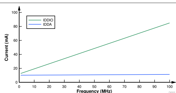
图 7-3. 电流与频率间的关系 - 内部 VREG
