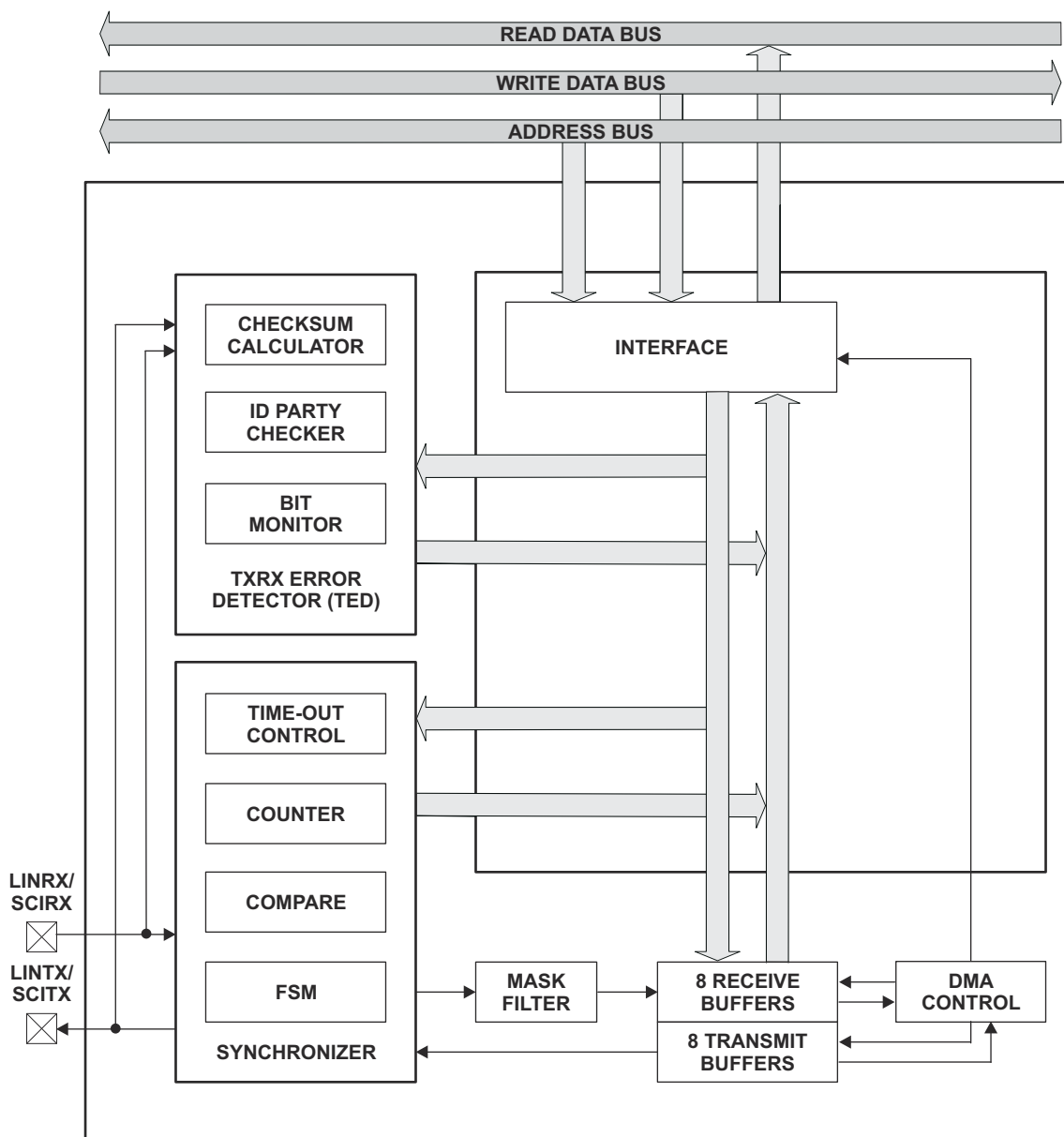
图 7-92. LIN 方框图
