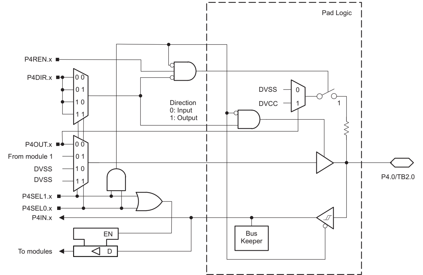
图 6-19. Port P4 (P4.0) Diagram
