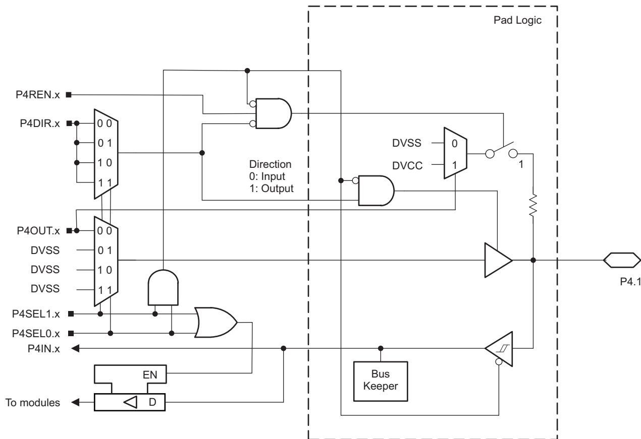
图 6-20. Port P4 (P4.1) Diagram
