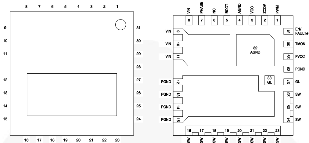
图 3. 引脚配置—俯视图和透视图
