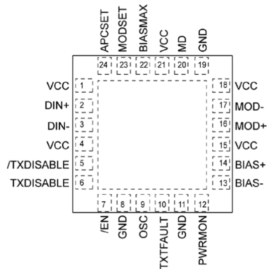
24-Pin QFN
