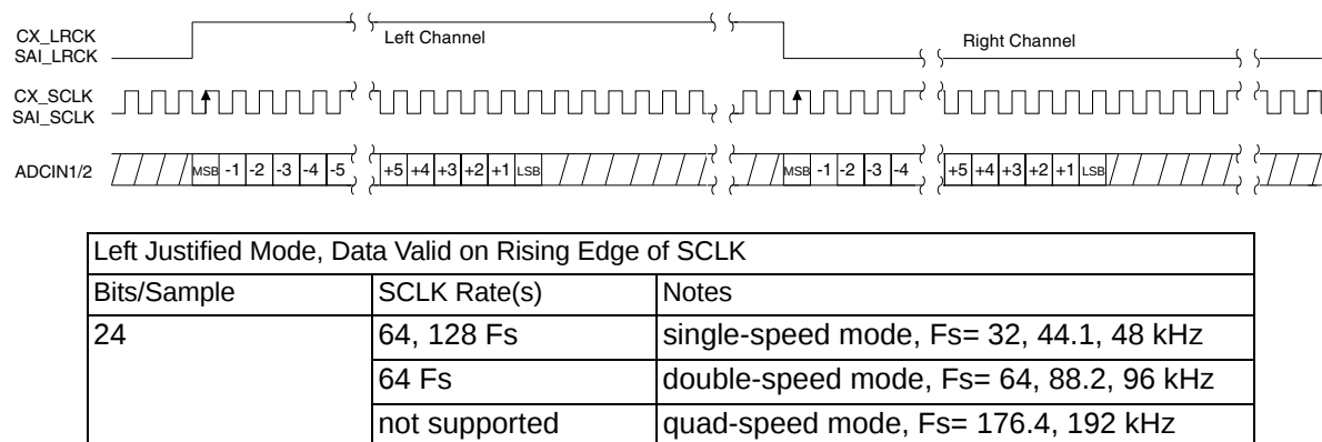
Figure 15. ADCIN1/ADCIN2 Serial Audio Format
