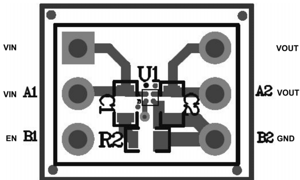
Top Layer
