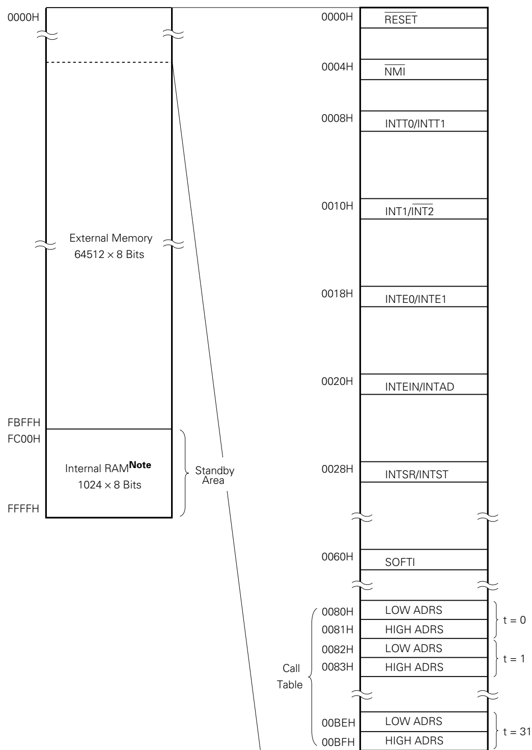
Fig. 2-3 μPD78C17 Memory Map
