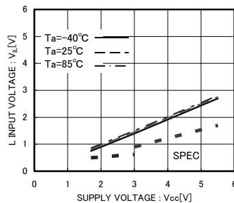
Fig.4 'L' input voltage V_{IL} (A0,A1,A2,SCL,SDA,WP)
