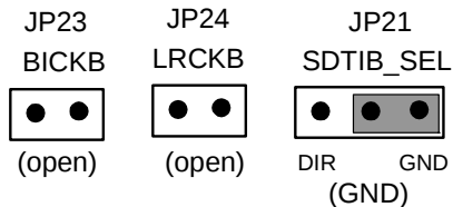
Figure 30. JP23 (BICKB), JP24 (LRCKB), JP21 (SDTIB_SEL)
