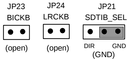
Figure 36. JP23 (BICKB), JP24 (LRCKB), JP21 (SDTIB_SEL)
