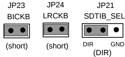
Figure 33. JP23 (BICKB), JP24 (LRCKB), JP21 (SDTIB_SEL)
