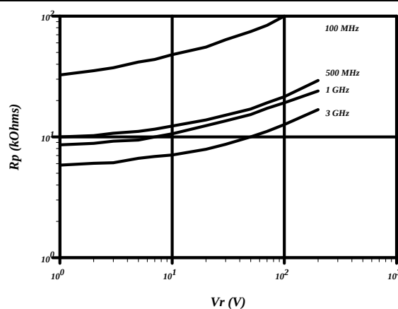
R_P VS V_R (UM7300)
