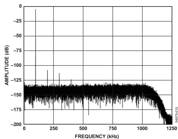
图14. 低功耗模式FFT, 100 kHz, -0.5 dB输入, 8×抽取
