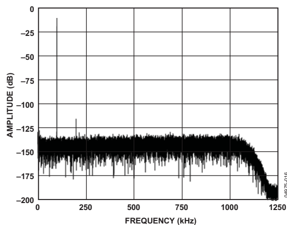
图15. 低功耗模式FFT, 100 kHz, -6 dB输入, 8×抽取
