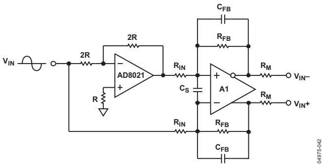
图53. 单端转差分
