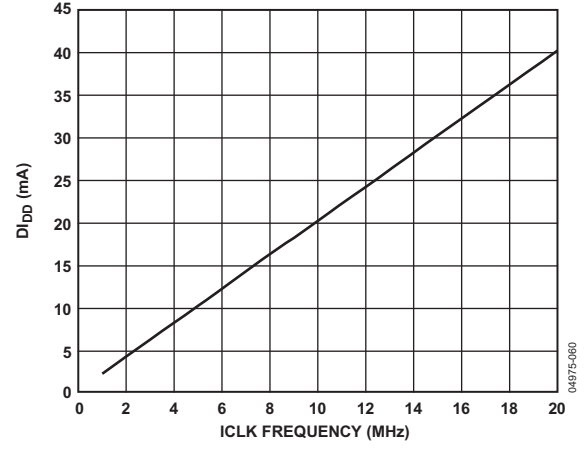
图39. 抽取× 256, DI_{DD} 与ICLK频率的关系( DV_{DD} = 2.5\text{ V} )
