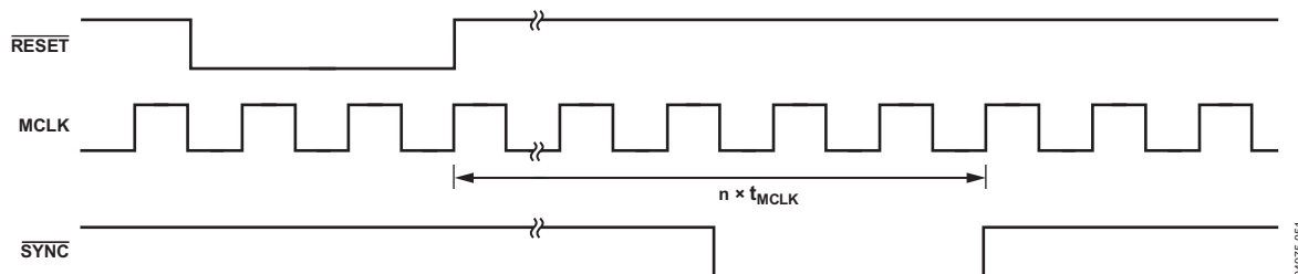
图44. AD7760在调制器输出模式下且CDIV= 0时，RESET与SYNC之间的相对时序
