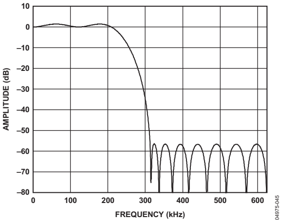
图58. 24抽头FIR滤波器频率响应
