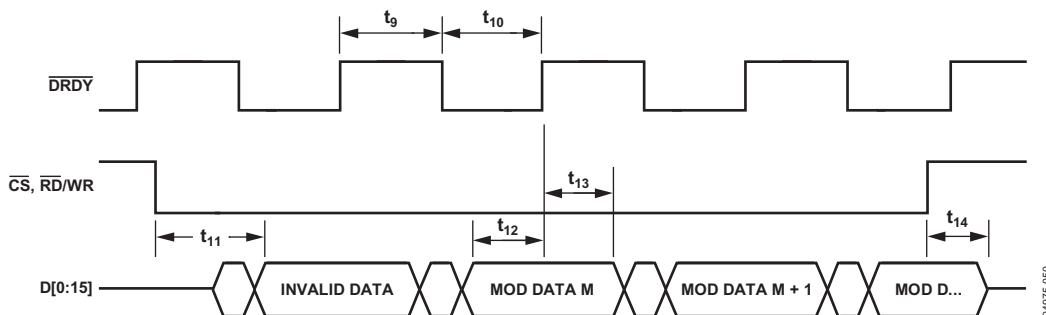
图43. AD7760调制器输出模式(CDIV= 1)且(CDIV= 0, n为偶数)
