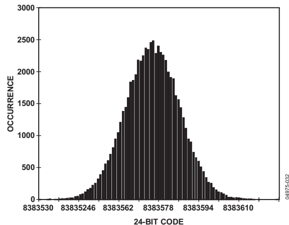
图32. 低功耗模式，24位直方图，256×抽取
