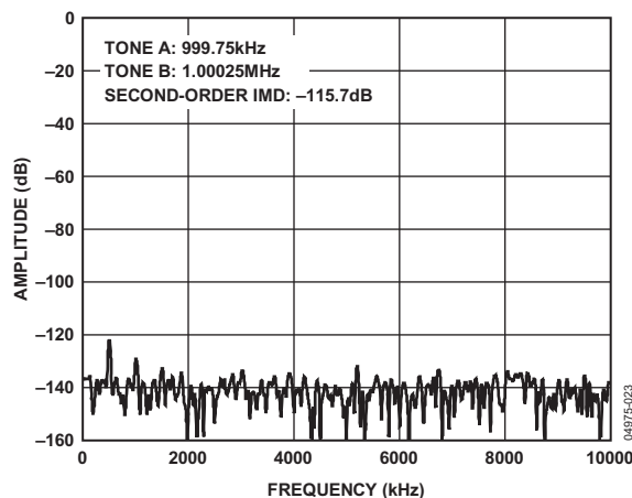
图22. 低功耗模式IMD, 1 MHz中心频率, 8×抽取
