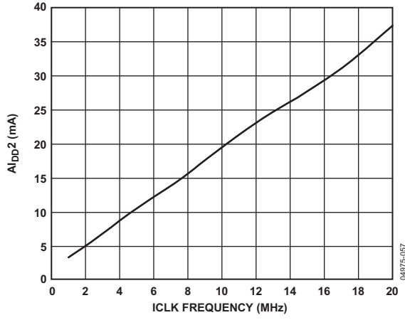
图36. AI_{DD2} 与ICLK频率的关系( AV_{DD2} = 5\text{ V} )
