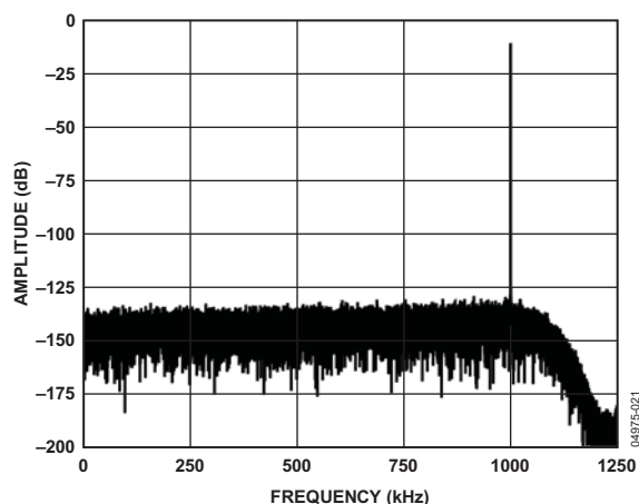
图20. 低功耗模式FFT, 1 MHz, -6 dB输入, 8×抽取
