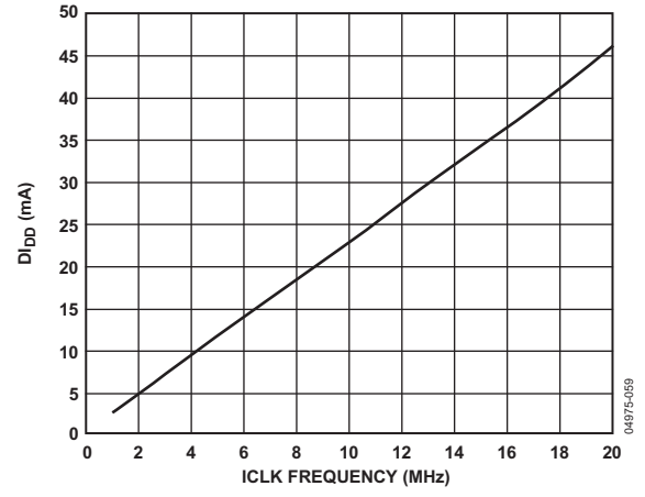
图38. 抽取× 32, DI_{DD} 与ICLK频率的关系( DV_{DD} = 2.5\text{ V} )
