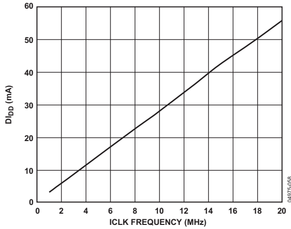
图37. 抽取× 8, DI_{DD} 与ICLK频率的关系( DV_{DD} = 2.5\text{ V} )
