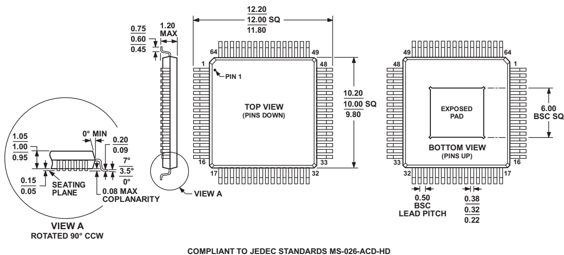
图59. 64引脚裸露焊盘、超薄四方扁平封装[TQFP_EP](SV-64-2) 尺寸(单位: mm)
