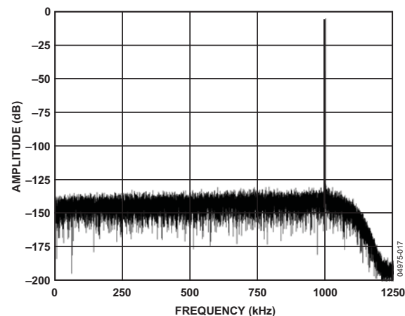
图16. 低功耗模式FFT, 1 MHz, -0.5 dB输入, 8×抽取
