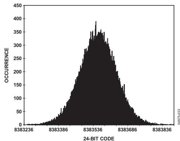
图33. 低功耗模式，24位直方图，8×抽取
