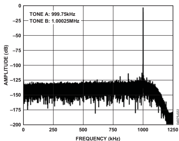
图21. 低功耗模式IMD, 1 MHz中心频率, 8×抽取
