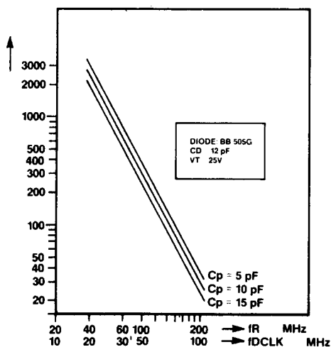
f) L/f-diagram
