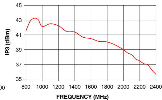
ZX60-2411BM+ IP3
