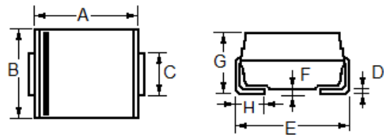
SMA
