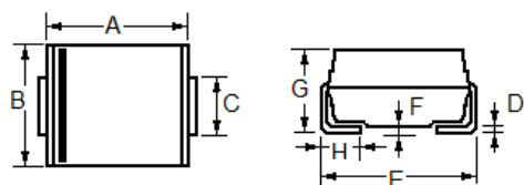
SMA
