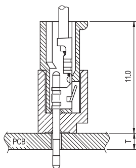
PCB ASS'Y
