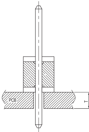
PCB ASS'Y
