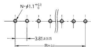
寸法表
