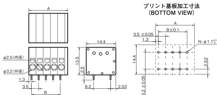
寸法表
