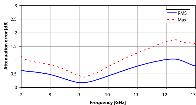
Attenuation Error
