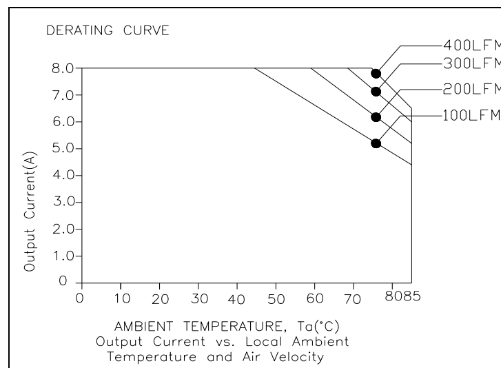
Figure 22. Vo = 7.5 V
