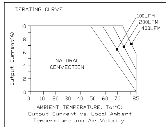
xRSB-40U03x
