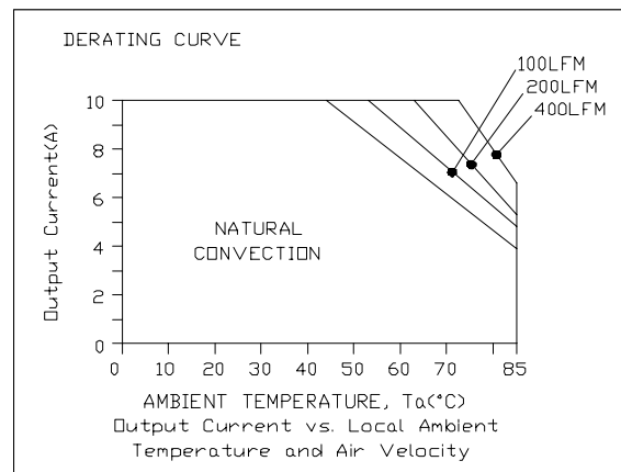
xRSB-40U03x
