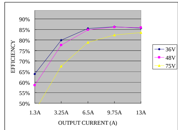
Vo=1.5 V
