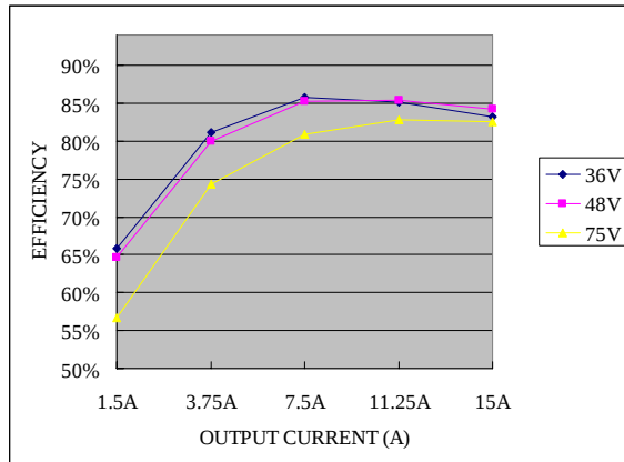
Vo=1.2 V
