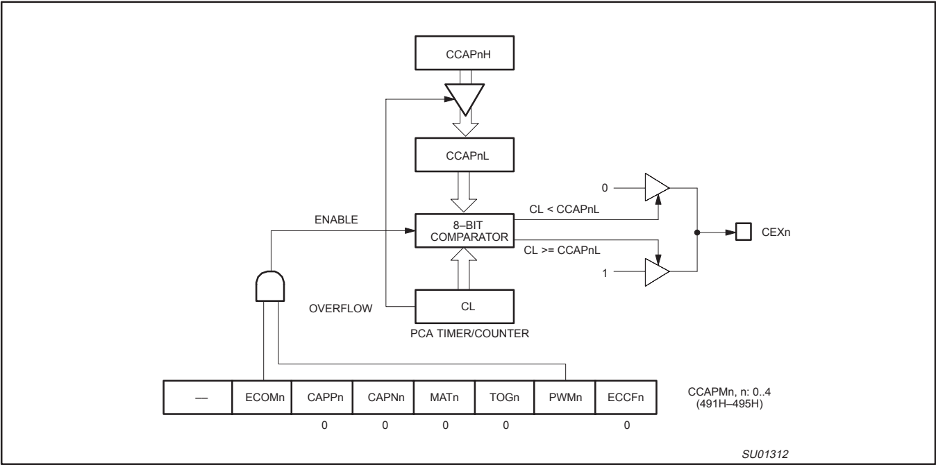
Figure 17. PCA PWM Mode
