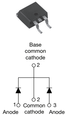
D 2 PAK
