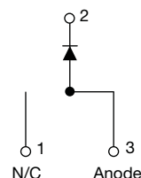
VS-8ETU04-1PbF
