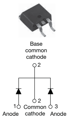
VS-30CTQ...SPbF
