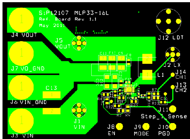
Fig. 9 - Top Layer
