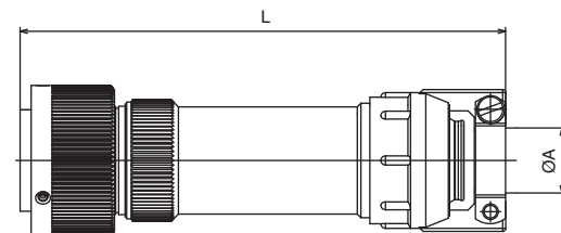
VBN6CF VBN6CFZ
