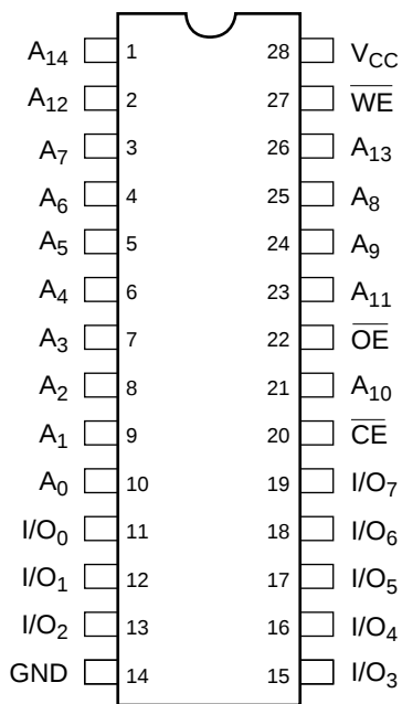
28-Pin SOJ
