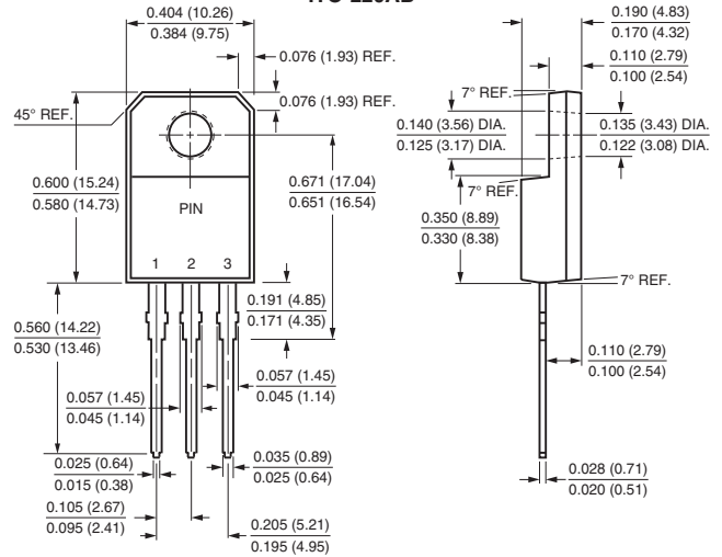
ITO-220AB
