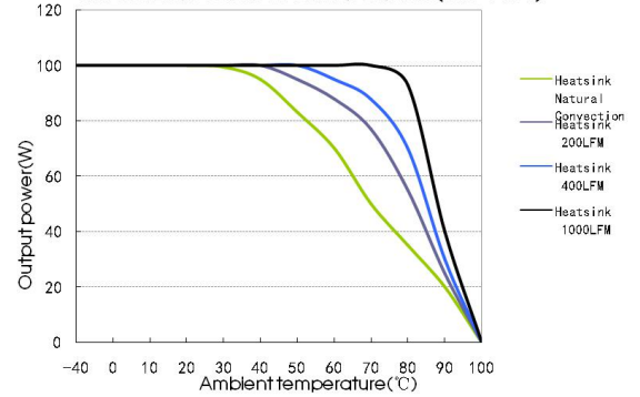
URF1D12QB-100WH Thermal Curves (Vin=110V)
